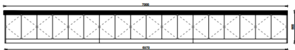
A面正视图
